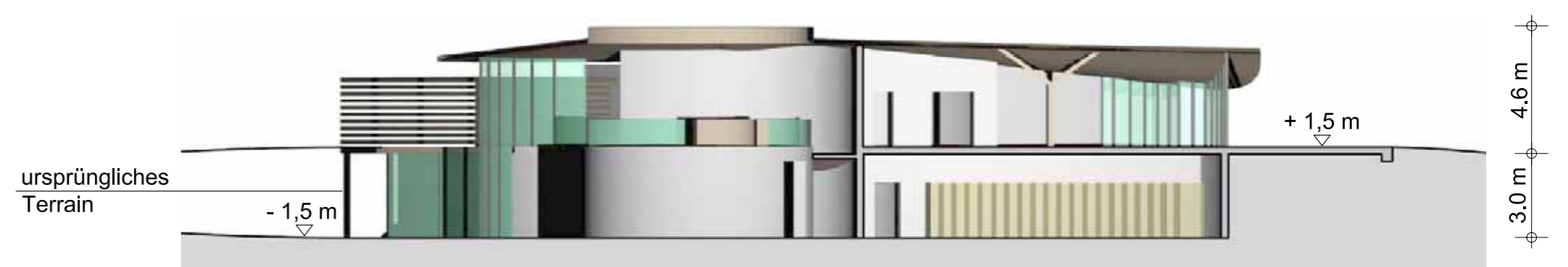
Schnitt M 1:200
