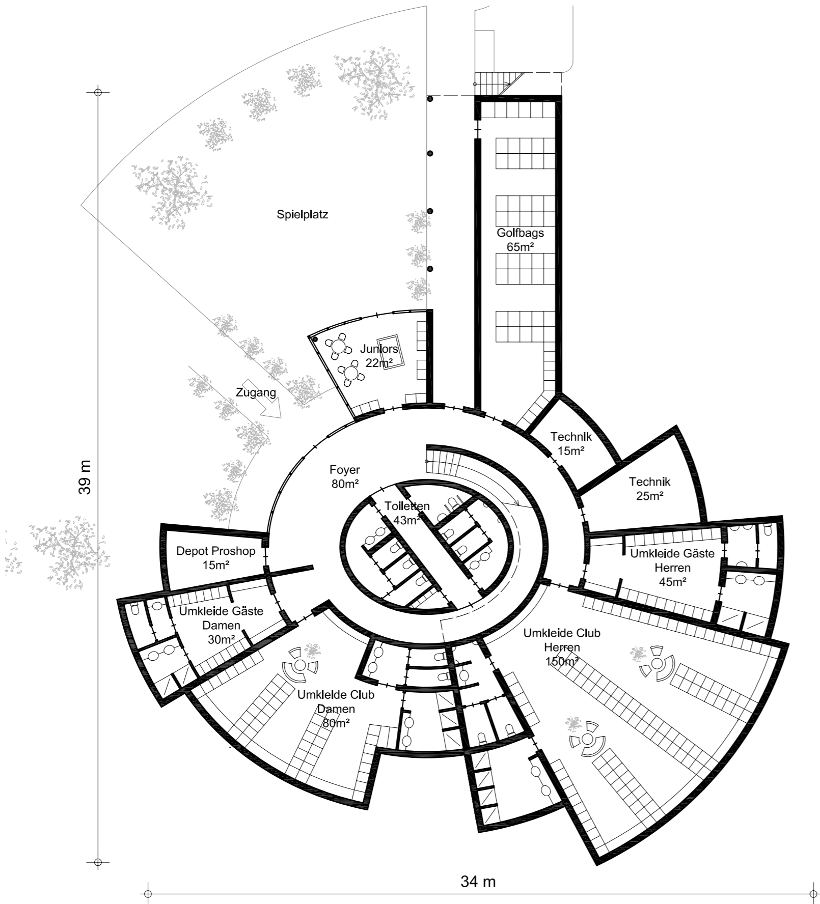
Grundriss Untergeschoss M 1:200
