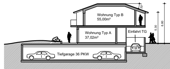
Haus I - Schnitt 1:200
