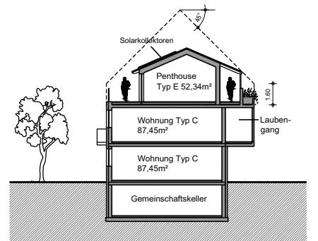
Haus III - Schnitt 1:200
