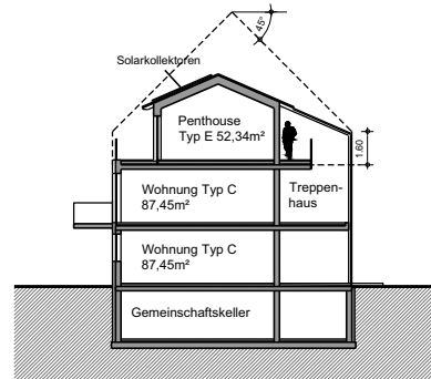
Haus II - Schnitt 1:200
