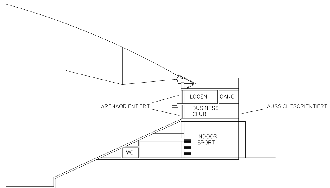
SCHNITT NORD
