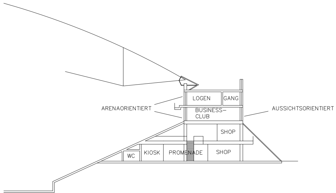
SCHNITT SÜD
