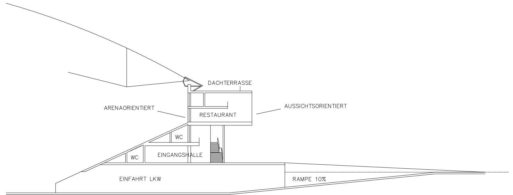
SCHNITT ECKBEREICH
