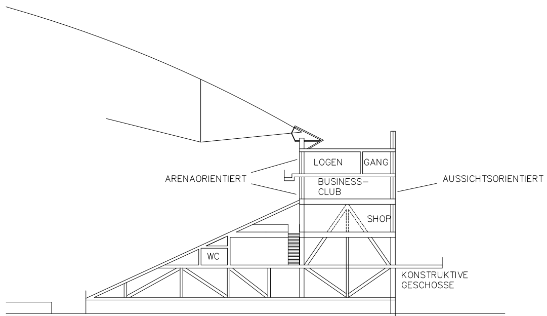
SCHNITT WEST
